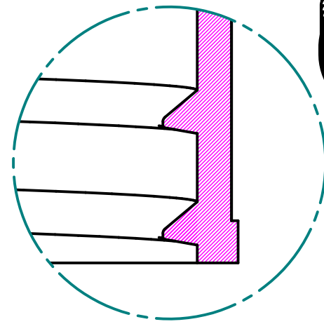
DETAIL B 5:1
